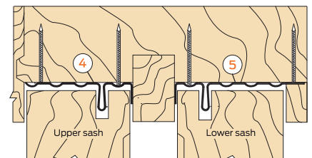
JAMB SECTION
